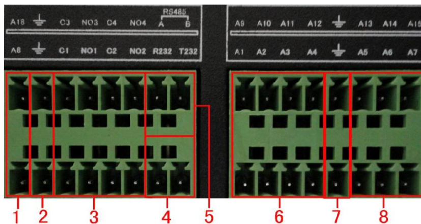
①⑥⑧报警输入 ②⑦地线 ③报警输出 ⑤RS485 ④RS232
